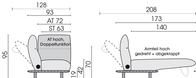
Seitenansicht 240DFH
