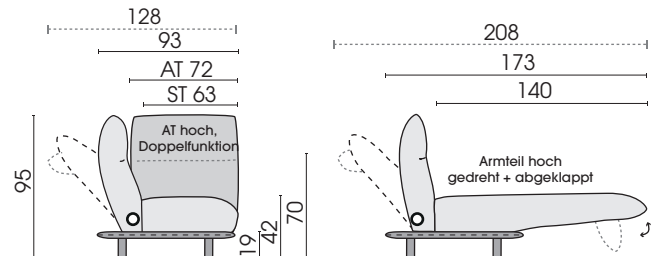
Seitenansicht M240DFH
